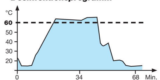
Temperaturkurve MoppWash® mit MEDIC Desinfektionsprogramm
